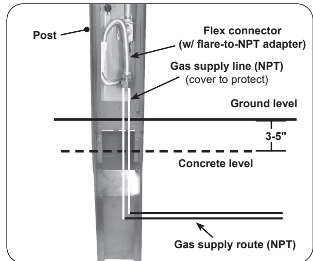
Fig. 30-3 Pour concrete & install post
